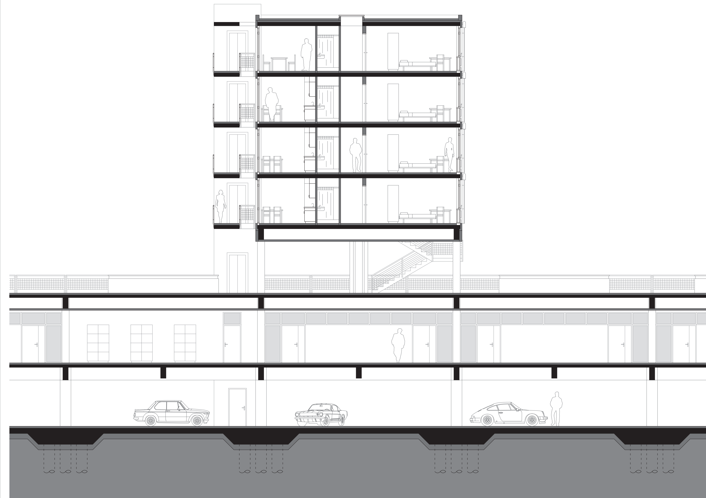
Coupe longitudinale type sur les circulations horizontales 1:100
