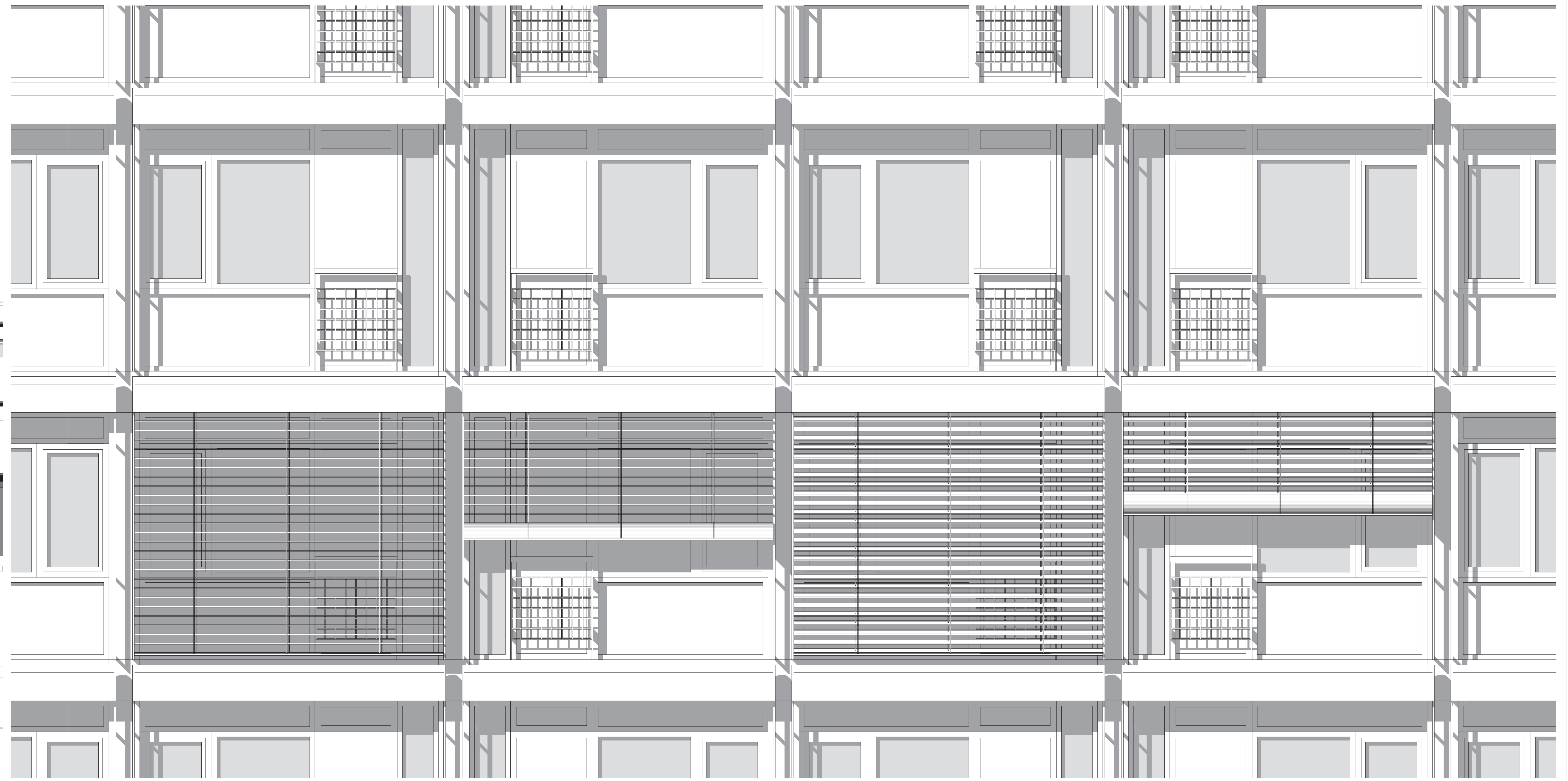
Façade est 1:20
