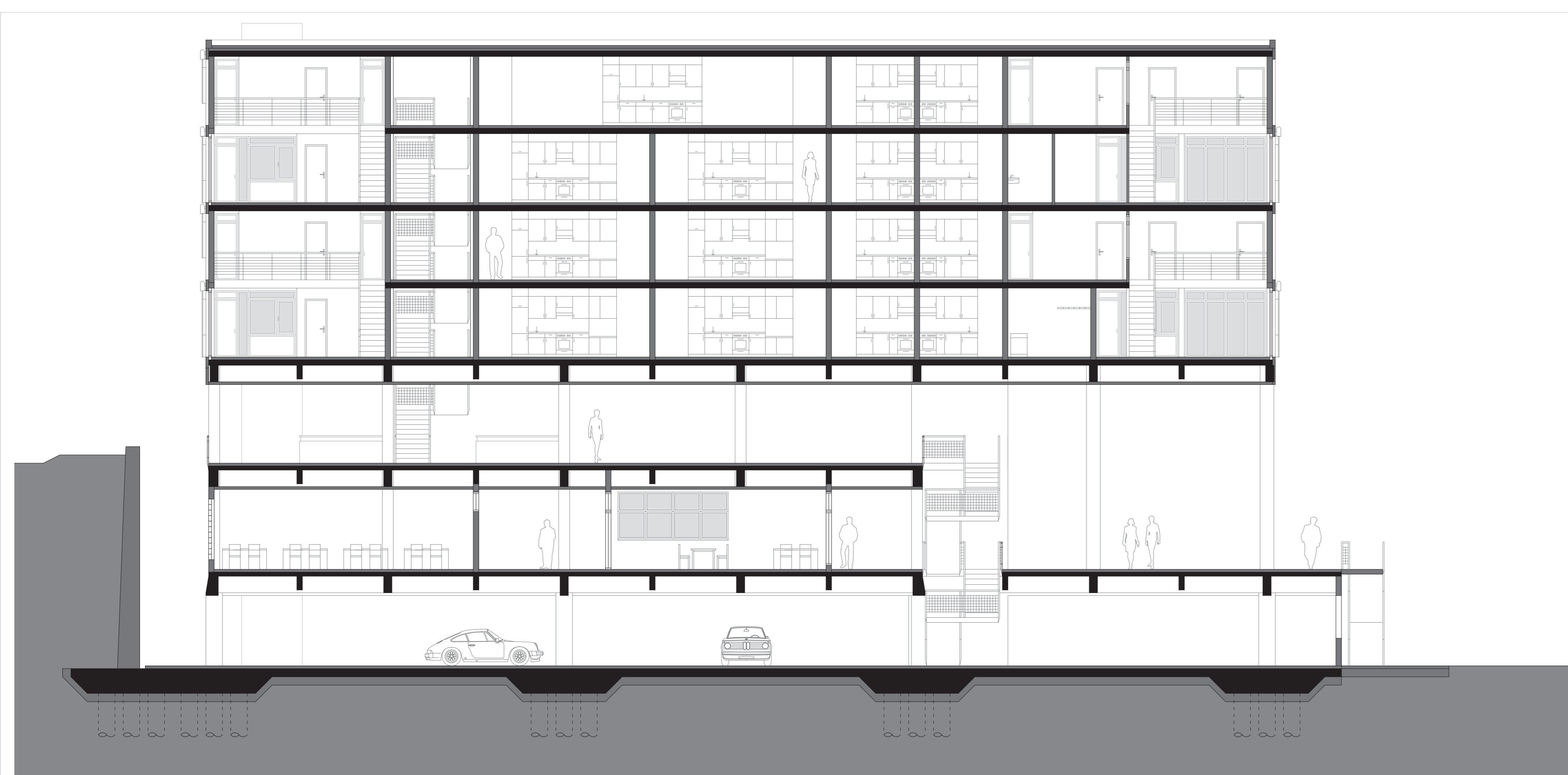
Coupe transversale type sur les espaces communautaires 1:100
