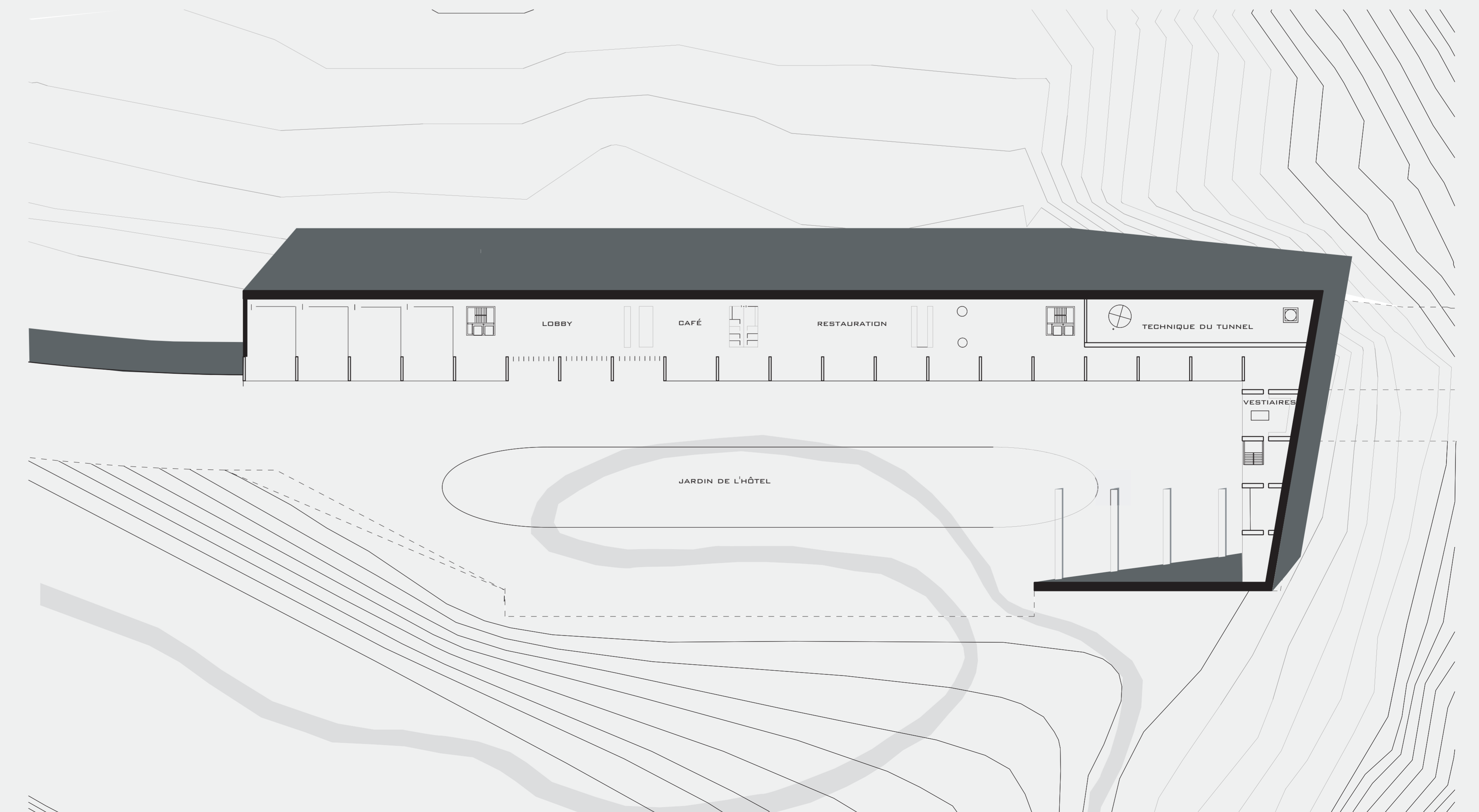
DIGUE - PLAN NIVEAU ENTRÉE, ÉCH. 1/500
