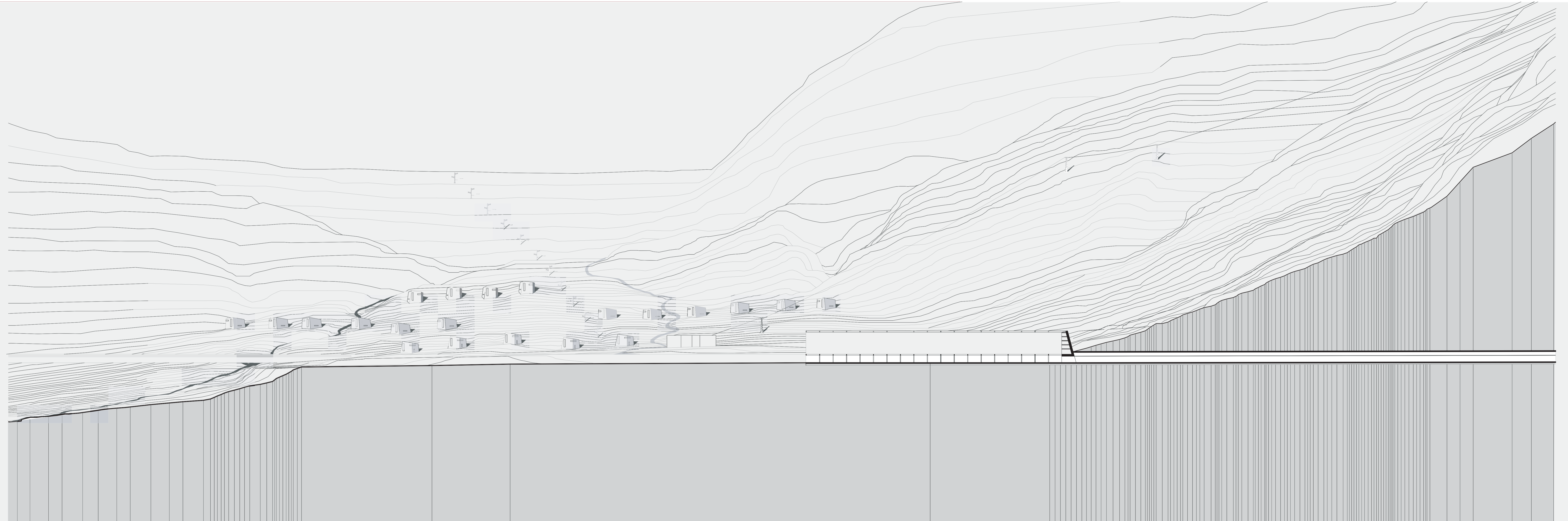
PRINCIPE STRUCTUREL DE LA DIGUE STRUCTURE ÉVOLUTIVE EN TROIS PHASES SELON LA PENTE ET LA VITESSE DES AVALANCHES
