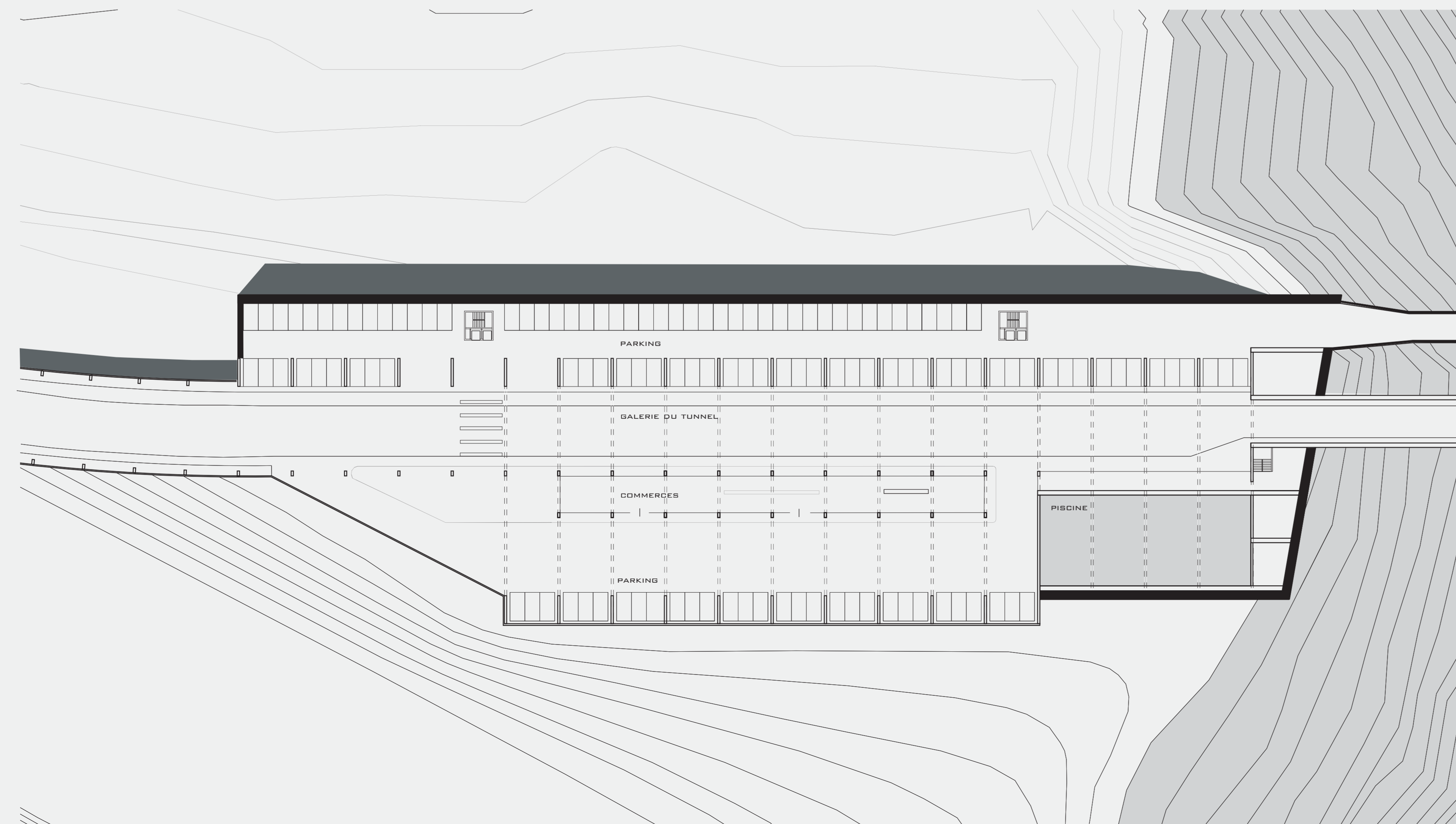
DIGUE - PLAN NIVEAU TUNNEL, ÉCH. 1/500
